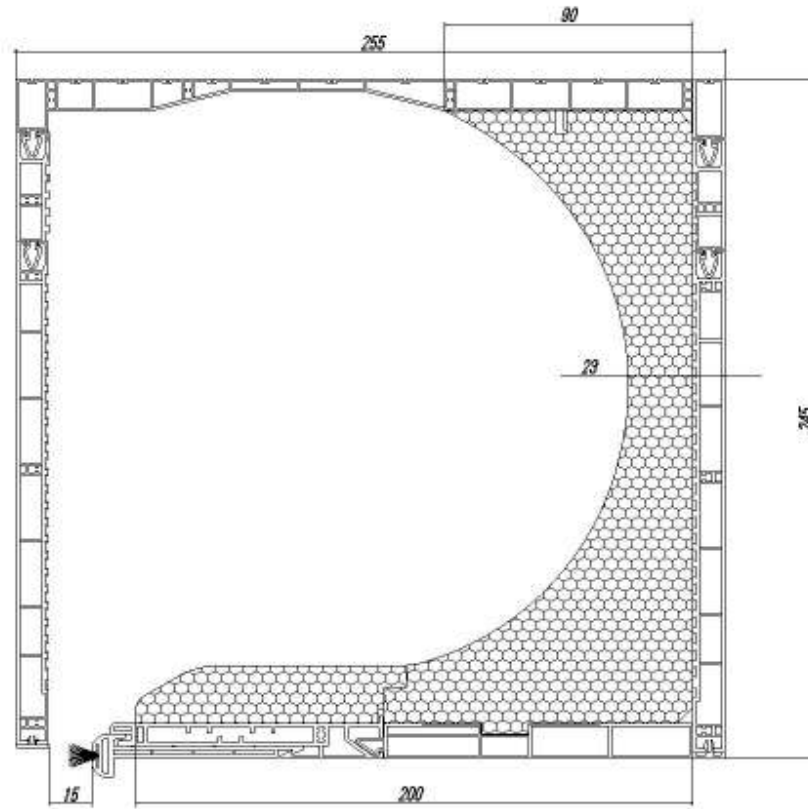
Bild 2 Schnittzeichnung
